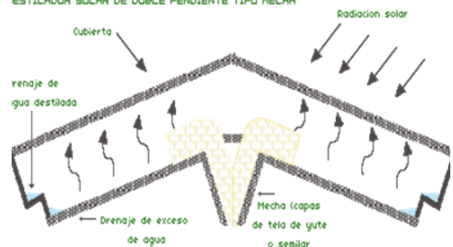
DESTILADOR SOLAR DE DOBLE PENDIENTE TIPO MECHA
